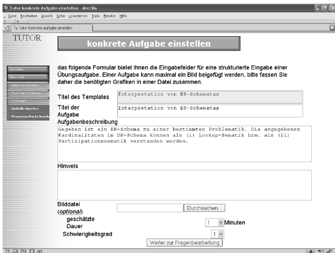
Abb. 1: Eingabemaske für das Einstellen einer Aufgabe
