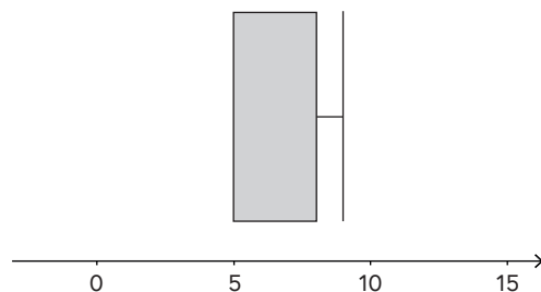
Abbildung 4: Ein degeneriertes Boxplot
