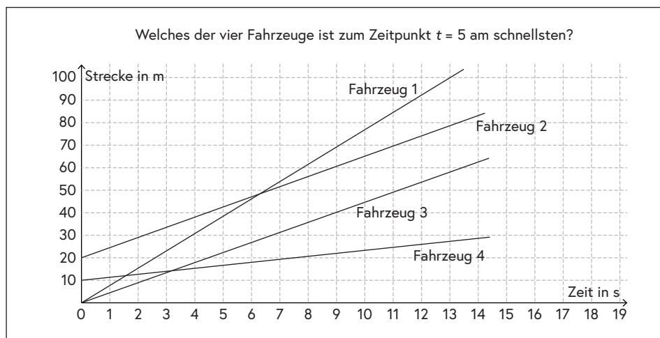
Abbildung 9: Zum Slope-Height-Fehler (Nitsch & Johlke, 2016, S. 705)
