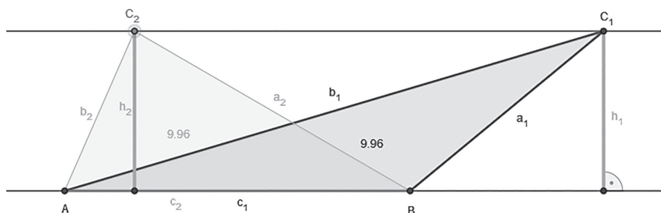
Abbildung 6: Zwei nicht kongruente, aber flächengleiche Dreiecke (Loher, n. d.)
