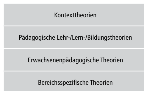
Abb. 1: Theorieebenen
