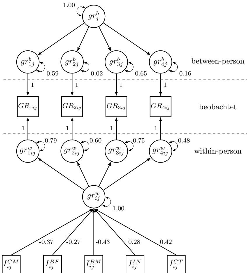
Abbildung 1: Pfaddiagramm der MCFA mit effektkodierten Indikatorprädiktoren
