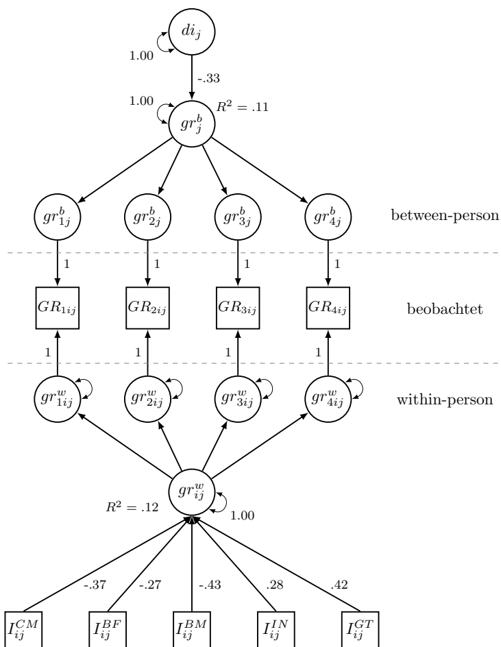
Abbildung 2: Pfaddiagramm der MLSEM
