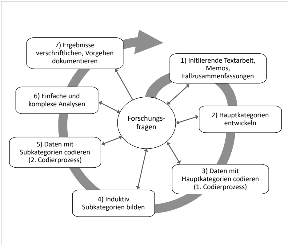
Abb. 9: Ablauf einer inhaltlich strukturierenden qualitativen Inhaltsanalyse in 7 Phasen (Kuckartz/ Rädiker 2022: 132)
