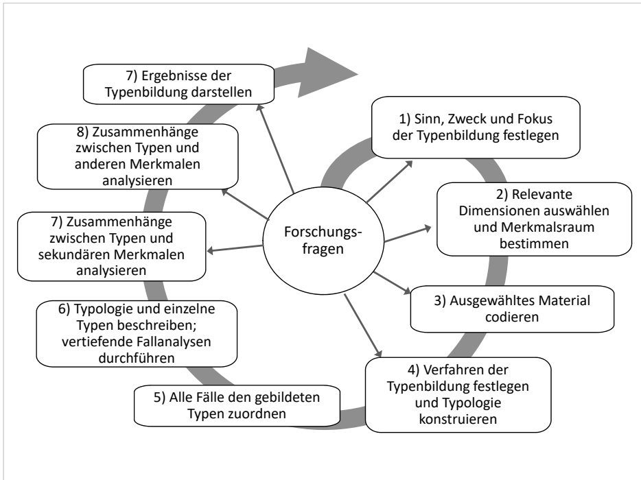
Abb. 11: Ablaufschema der typenbildenden qualitativen Inhaltsanalyse (Kuckartz/ Rädiker 2022: 186)
