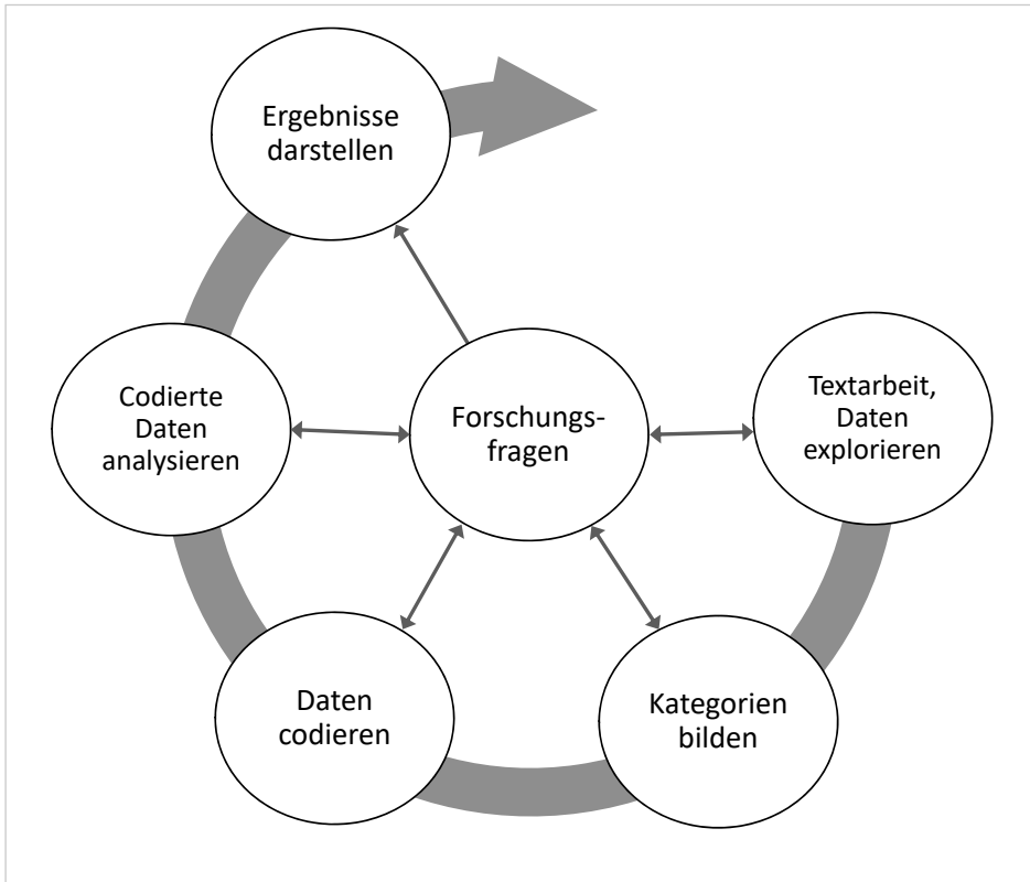
Abb. 8: Allgemeines Ablaufmodell qualitativer Inhaltsanalysen (Kuckartz/ Rädiker 2022: 106)
