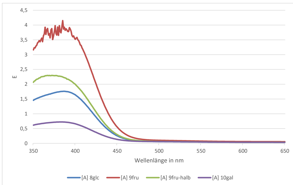
Abbildung 139: Phenylhydrazin-Werte aus den gelben Lösungen, 1 mm-Küvette
