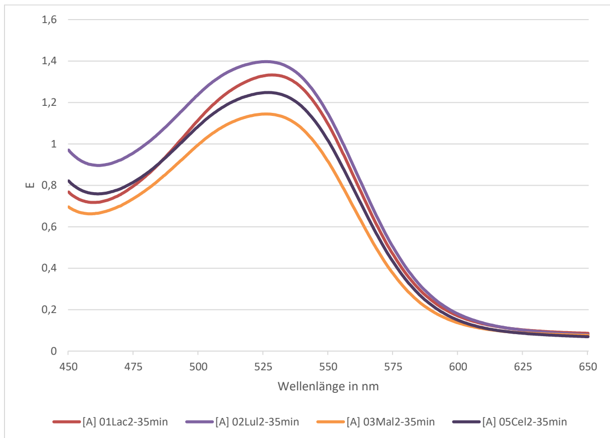
Abbildung 80: Wöhlk-Probe mit Zuckerlösungen ( \omega = 1\% )
