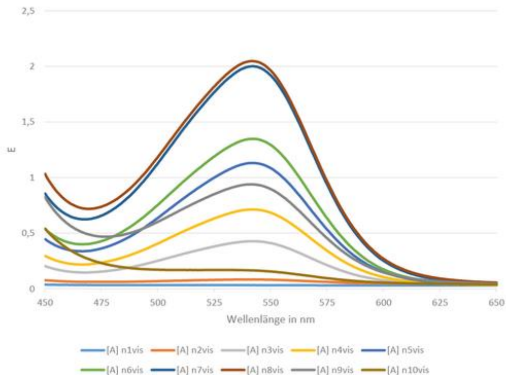
Abb. 4: Absorption der Proben 1 bis 10 im Vis-Bereich.
