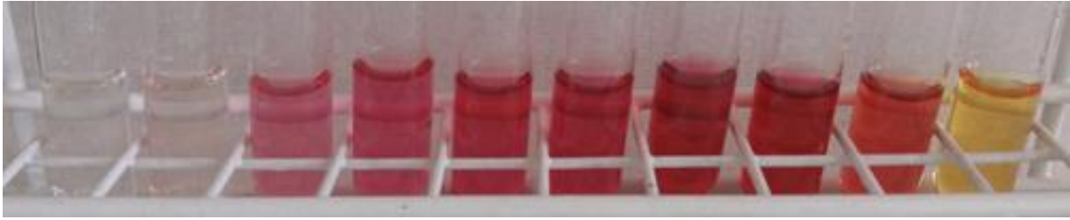
Abb. 3: Die zehn Proben aus dem Nickerson-Experiment mit pH 11,7 (ganz links), bis pH 13,29 (ganz rechts). Der optimale pH-Wert liegt bei 12,8 (fünfte Probe von links).
