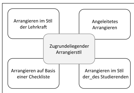
Abbildung 2: Zugrundeliegender Arrangierstil
