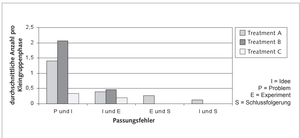
Abb. 12: Passungsfehler
