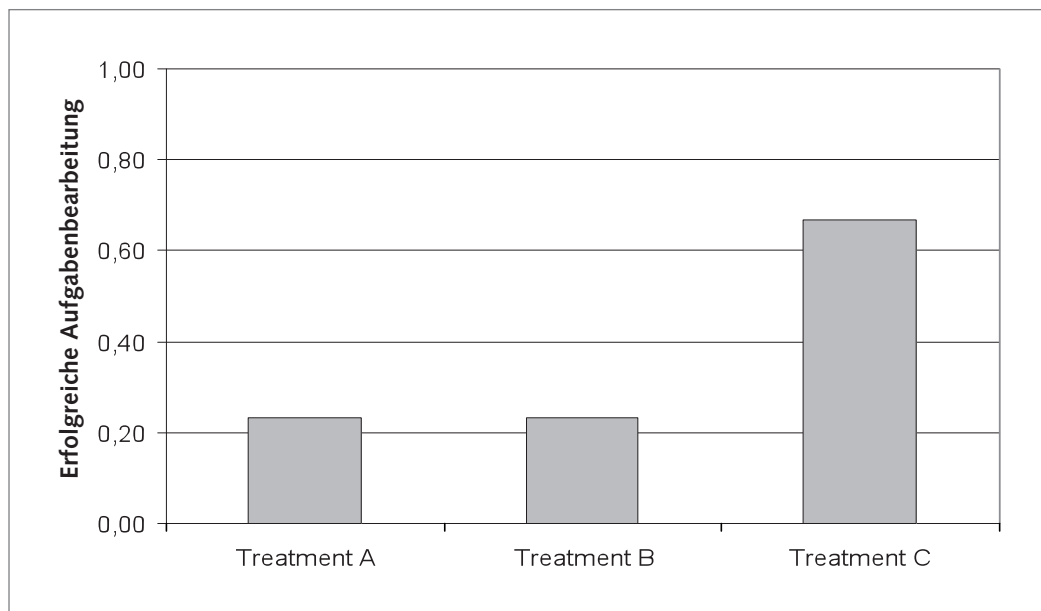
Abb. 10: Erfolgreiche Aufgabenbearbeitung
