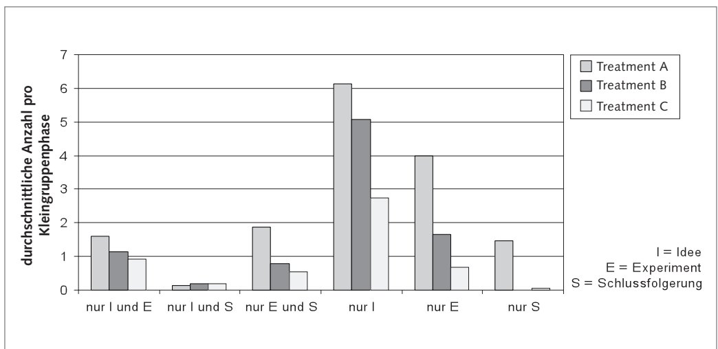
Abb. 11: Auslassungsfehler
