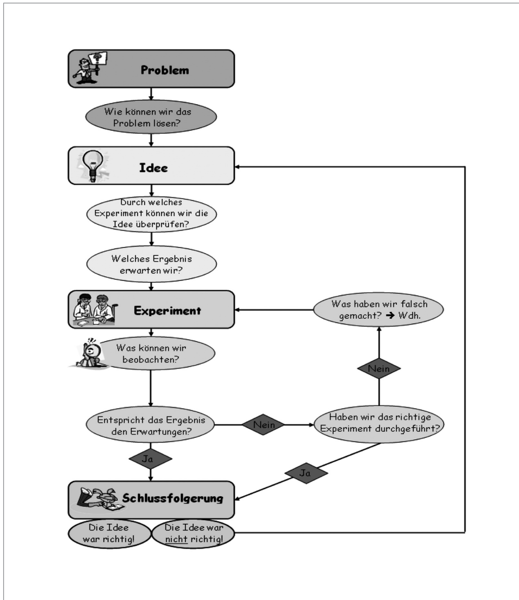
Abb. 1: Strukturierungshilfe
