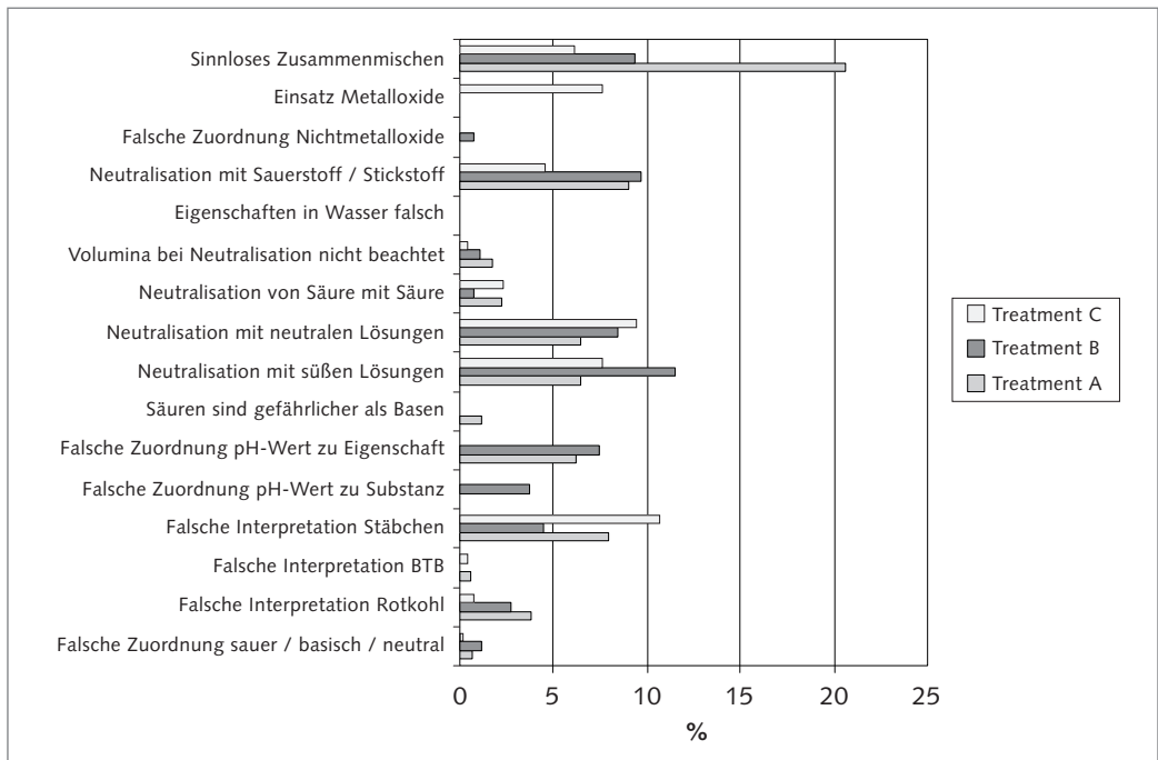
Abb. 8: Inhaltliche Fehler
