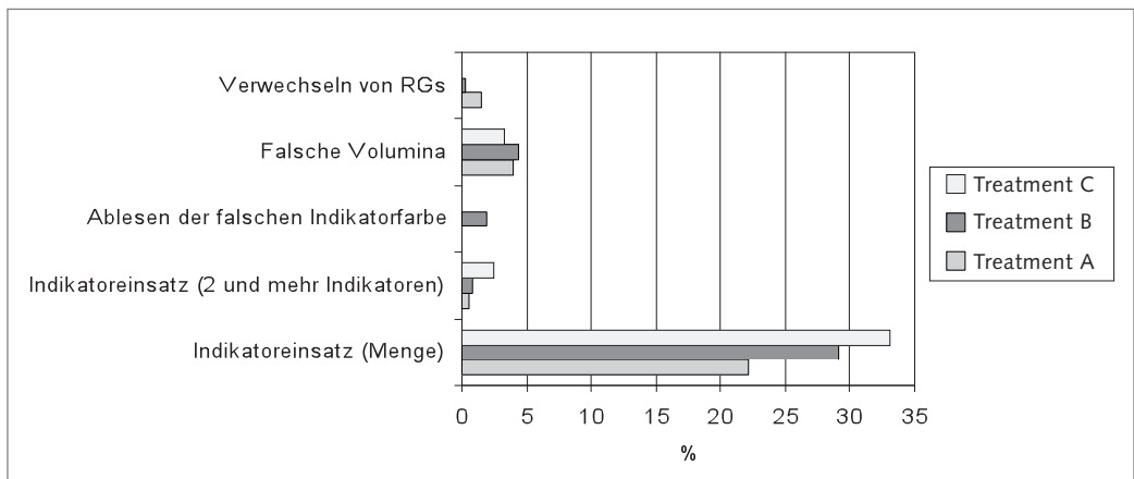
Abb. 9: Manuelle Fehler
