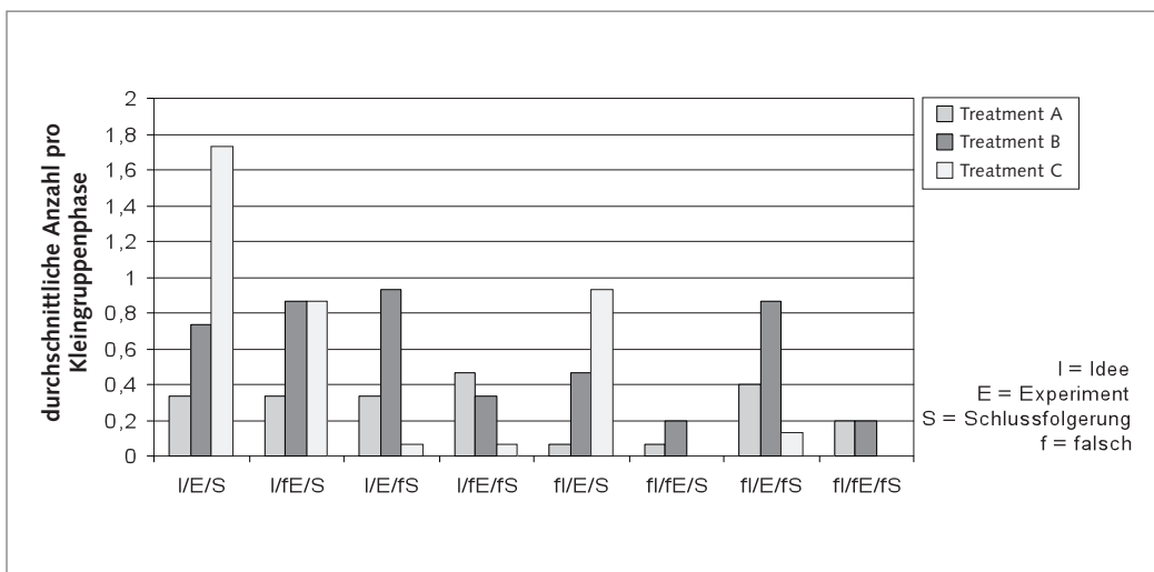
Abb. 13: Problemlöseprozess
