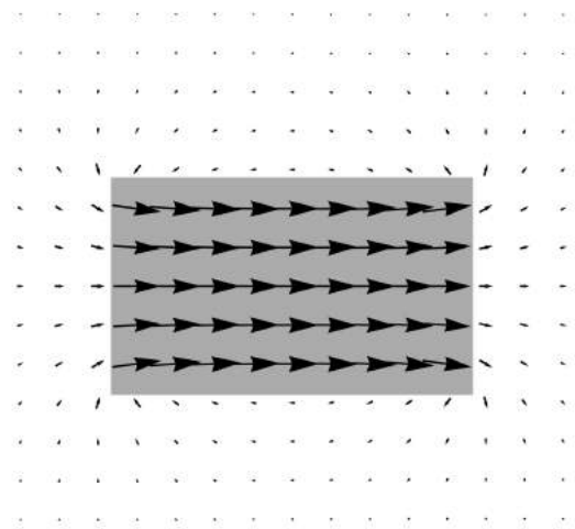
(b) Verlauf des \vec{B} -Feldes im Schnitt z = 0 durch den Permanentmagneten.
