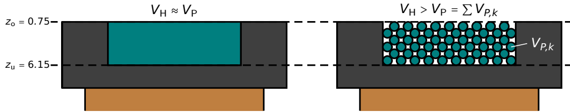
Abbildung 5.10: Vergleichende Darstellung der Füllung des Probenhalters bei blockförmigen und flüssigen Proben (links) und Proben in granular Form (rechts).
