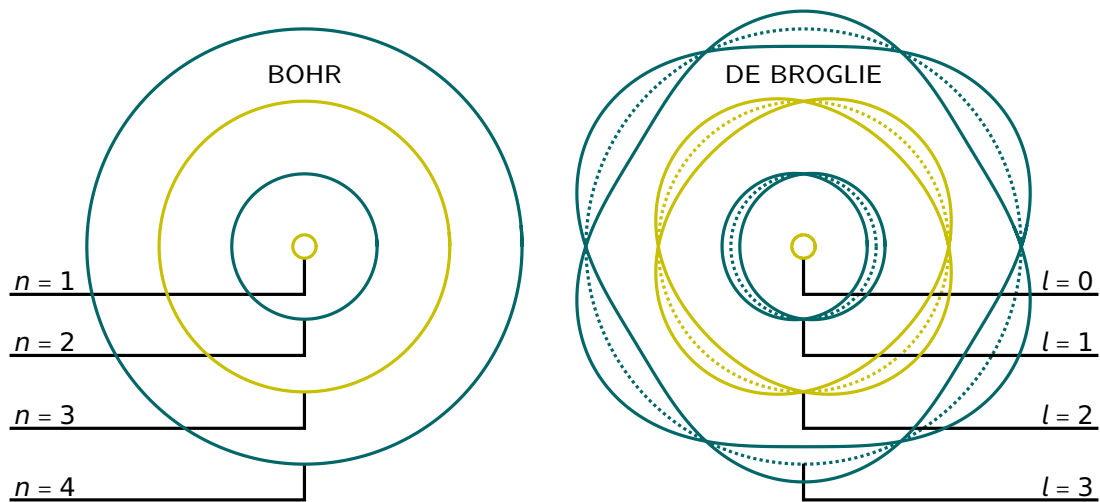
Abbildung 4.33: Darstellung kreisförmiger Elektronenzustände im Bohrschen Atommodell sowie der Erweiterung nach de Broglie durch Zuordnung stehender.
