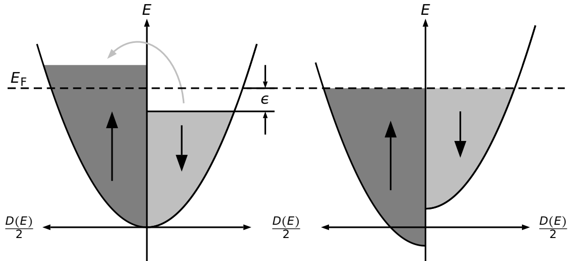
Abbildung 4.59: Visualisierung des Stoner-Modells zur Beschreibung der Entstehung spontaner Magnetisierungen und ferromagnetischer Zustände nach [Nol09, S. 185]. Der zunächst aufzuwendenden kinetische Energiebeitrag kann durch den Gewinn potentieller magnetischer Energie ausgeglichen werden.
