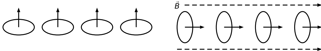
Abbildung B.3: Darstellung der Ursache für die magnetokristalline Anisotropie bei Spinausrichtung und Umoorientierung der Elektronenverteilung durch Spin-Bahn-Kopplung.
