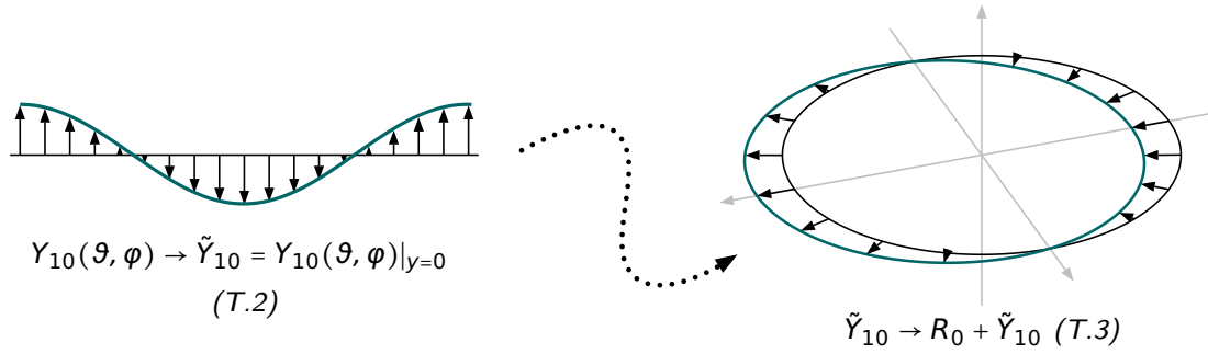
Abbildung 4.21: Visualisierung der Wellenfunktion \Psi_{210}(r, \vartheta, \varphi) ( p -Welle) nach Transformation (T.2) und (T.3), d. h. nach Schnitt durch die xz -Ebene und Transformation auf den Kreis mit Radius R_0 .
