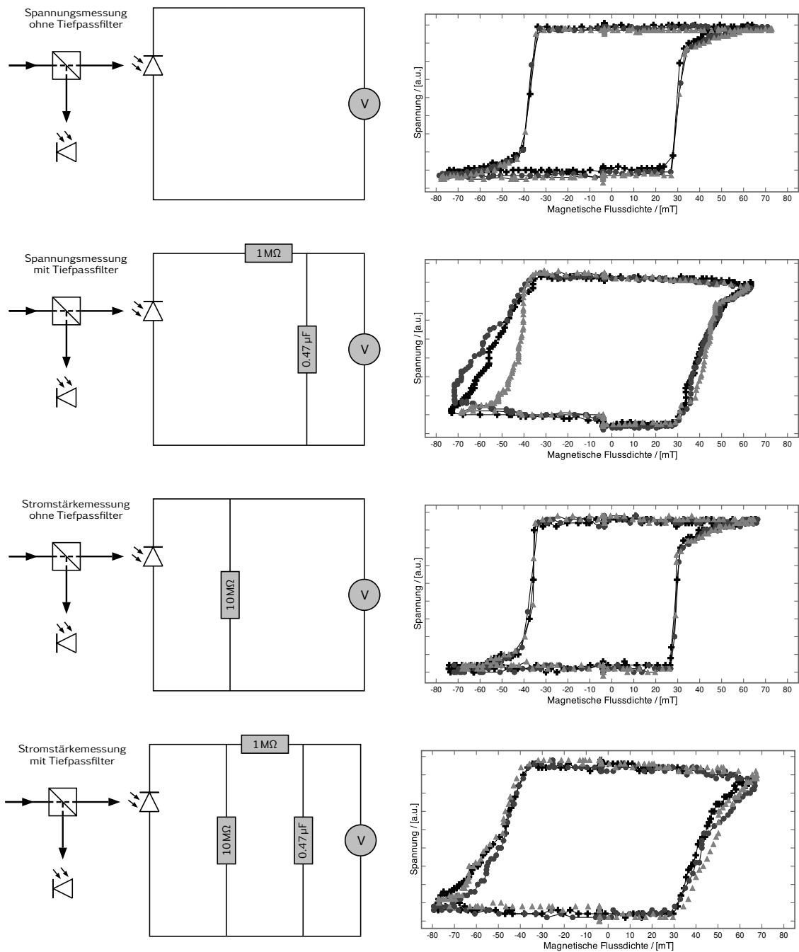
Abbildung 5.23: Messergebnisse der magnetischen Hysteresis einer Co/Pt-Probe mit mikrooptischer Bank und einer Photodiode. Zur Darstellung der Reproduzierbarkeit werden pro Versuchsaufbau drei Messungen durchgeführt und angegeben.
