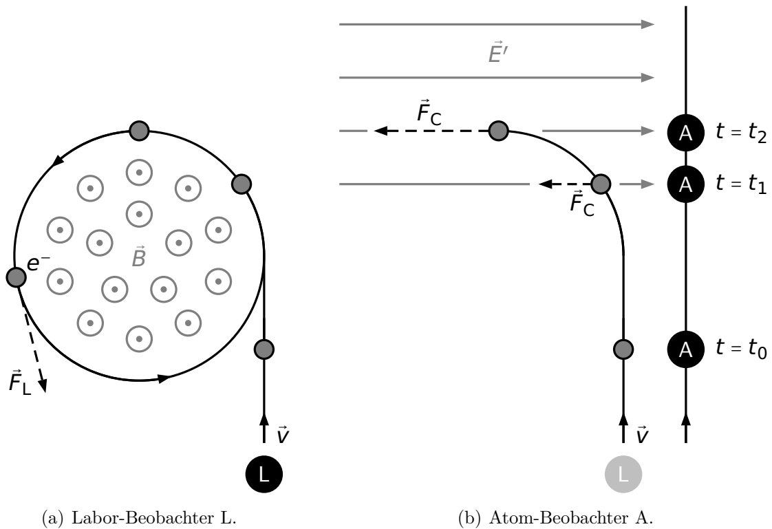
Abbildung 4.14: Schematische Darstellung des Gedankenexperiments zur Äquivalenz des \vec{B} - und \vec{E} -Feldes. Der Wechsel des Bezugssystems und die Betrachtung eines geladenen Teilchens im magnetischen bzw. elektrischen Feld ermöglicht die Transformation der Felder.
