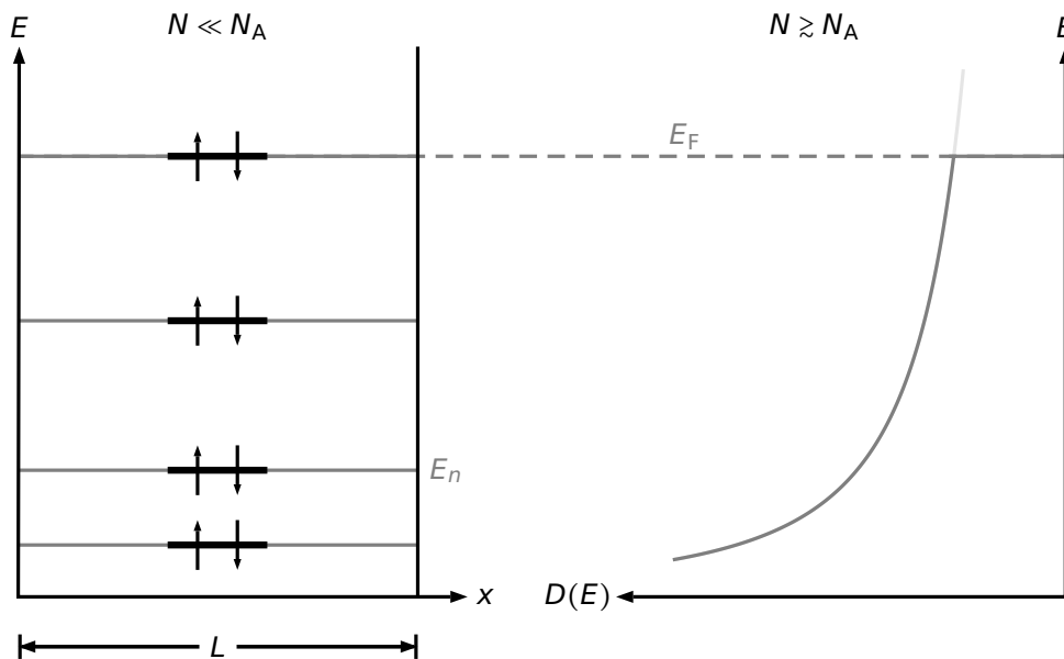
Abbildung 4.48: Vergleichende Darstellung der diskreten besetzten Energieniveaus für N \ll N_A sowie bei großen Teilchenzahlen N \gtrsim N_A im Übergang zur kontinuierlichen Zustandsdichte bei T=0 nach [Dem10, S. 458].
