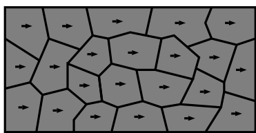
Abbildung 4.16: Schematische Darstellung des Modells der Weiss'schen Bezirke für unterschiedliche Grade der Magnetisierung. Bei der didaktischen Modellierung wird die Korrelationslänge und die Änderung der Größe der Weiss'schen Bezirke nicht explizit gemacht.
