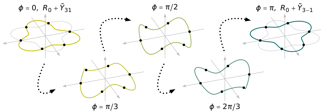
Abbildung 4.24: Darstellung des Erhaltes von sechs Knotenpunkten am Beispiel der Wellenfunktion \Psi_{431} (f-Welle) nach Transformation (T.4) bei Variation der Phase \varphi . Neben der Aufenthaltswahrscheinlichkeit ist auch die Anzahl der Knotenpunkte unter dieser Transformation invariant.
