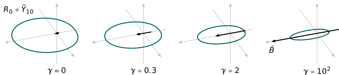
Abbildung 4.54: Qualitative Darstellung von Schnitten durch die Wellenfunktionen Y_{10} und Y_{11} mit linearer Ausrichtung eines magnetischen Felds und unterschiedlicher Stärke nach [Rös84, S. 35]. Bei extrem starken Magnetfeldern ( \gamma > 0 ) zeigt sich ein erheblicher Einfluss des Magnetfeldes auf die Gestalt des Atomorbitals.
