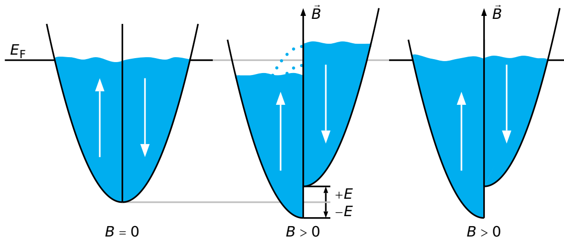
Abbildung 4.56: Modellierung der Verschiebung der Zustandsdichte D(E) durch Änderung der Energie in der Analogie als Wassermmodell. Die Analogie zur quantenmechanischen Größe der Zustandsdichte ermöglicht den Aufbau von Vorstellungen bei Gleichsetzung von Wassermolekülen und möglichen Zuständen.
