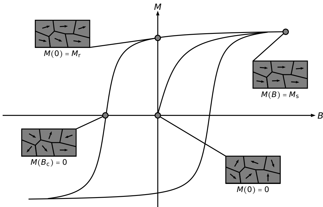
Abbildung 4.17: Schematische Darstellung der Weisschen Bezirke in Verbindung mit einer ferromagnetischen Hystereseurve. Die gemeinsame Visualisierung verbindet die formale BM -Kurve mit der ikonischen Darstellung der ferromagnetischen Domänen.
