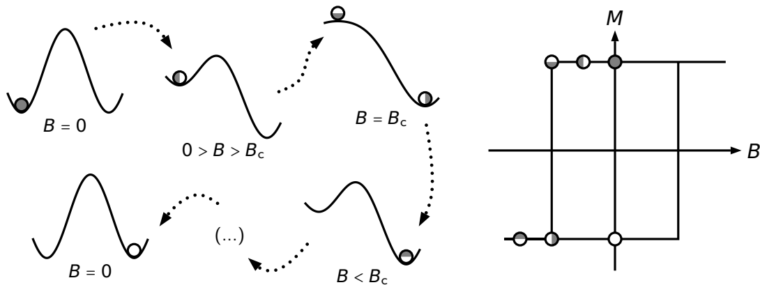
Abbildung B.4: Visualisierung der Abhängigkeit der Magnetisierung \vec{M} von der magnetischen Flussdichte \vec{B} für eine singuläre Domäne nach dem Stoner-Wohlfarth-Modell bei Ausrichtung des äußeren Magnetfeldes parallel zur leichten Achse der magnetokristallinen Anisotropie und Abbildung der zu unterschiedlichen Zuständen gehörigen Potentialzustände.
