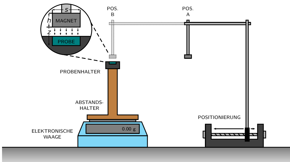
Abbildung 5.8: Versuchsaufbau der Magnetismus zur quantitativen Bestimmung der magnetischen Volumensuszeptibilität dia- und paramagnetischer Proben.
