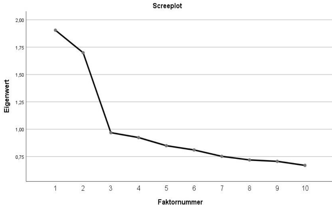
Abb. 3. Eine Analyse des Screeplots gibt starke Hinweise auf zwei unterliegende Faktoren in der Datenstruktur. Zum einen ist zu sehen, dass nur zwei Eigenwerte einen Wert von mehr als 1.00 besitzen, zum anderen bricht der Screeplot bei einem dritten Faktor stark. Auch dargestellt ist die nahezu gleichgroße Aufklärungsmächtigkeit der beiden ersten Faktoren: beide haben ähnlich hohe Eigenwerte.
