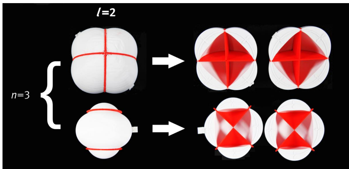
Abb. 14. Haptische Modelle der Wellenfunktionen eines Elektrons im Wasserstoffatom, die nur Knotenlinien im Radialteil haben (also l = n - 1 ). Links sind die Modelle geschlossen und die Außenseite ist zu sehen; rechts sind die Modelle geöffnet und das Innenleben wird sichtbar, wobei die roten Flächen die Knotenflächen sind. Die Schnittflächen entsprechen den Chladnischen Klangfiguren auf einer Rundplatte, die nur aus azimuthalen Knotenlinien bestehen. Die Entartung der d -Wellenfunktionen ist nur im dreidimensionalen sichtbar – die Schnitte sind in beiden Wellen Knotenlinien in einem Winkel von 90^\circ .
