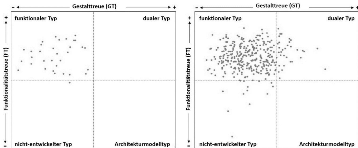
Abb. 7. Verteilung der Teilnehmenden im Bereich der Hochschullehrer/-innen (links) und Lehrer und Lehrerinnen (rechts) an der Onlineumfrage zu Modellvorstellungen auf den Quadranten der vier Typen mentaler Modelle . Es ist zu sehen, dass nahezu alle Teilnehmenden im oberen linken Quadranten aufzufinden sind.
