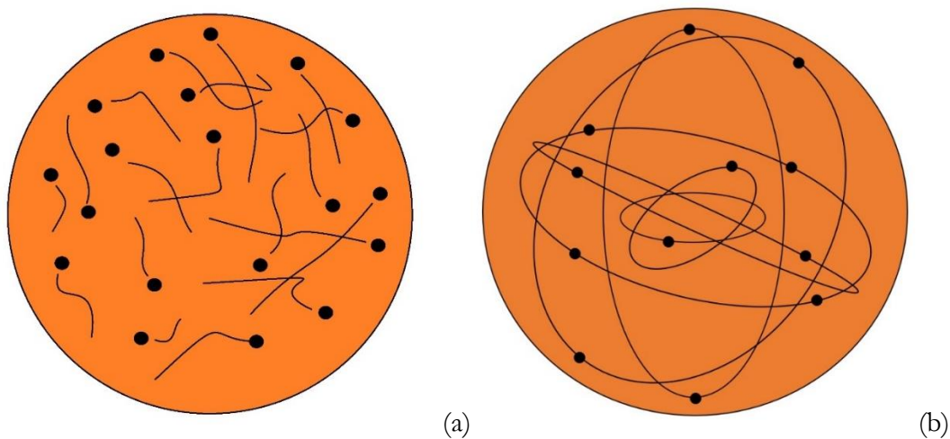
Abb. 9. Thomsons bekannteste Ansätze, das Atom zu beschreiben. Zunächst vermutete er, dass tausende Korpuskeln (Elektronen, schwarz) in einer masselosen positiv geladenen Hülle (orange) herumschwirrten (a), später schärfte er dieses Modell jedoch dahingehend aus, dass er annahm, die Elektronen würden auf unzähligen Ringen um den Mittelpunkt des Atoms rotieren, wobei die Anzahl der Elektronen auf den Ringen Aufschluss über die chemischen Eigenschaften geben sollten (b). Reproduziert nach THOMSON (1903).
