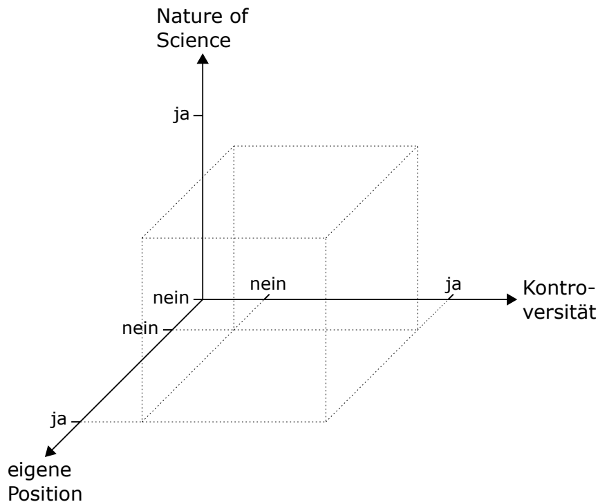
Abbildung 8.19: dreidimensionaler Merkmalsraum
