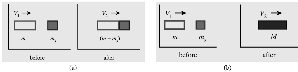
Abbildung 3.5: (a) Stoßprozess zur Definition der Masse (Atkin 2015, S. 48, Abb. 1) (b) relativistische Beschreibung eines Stoßprozesses zur Definition der Masse (ebd., S. 50, Abb. 5)
