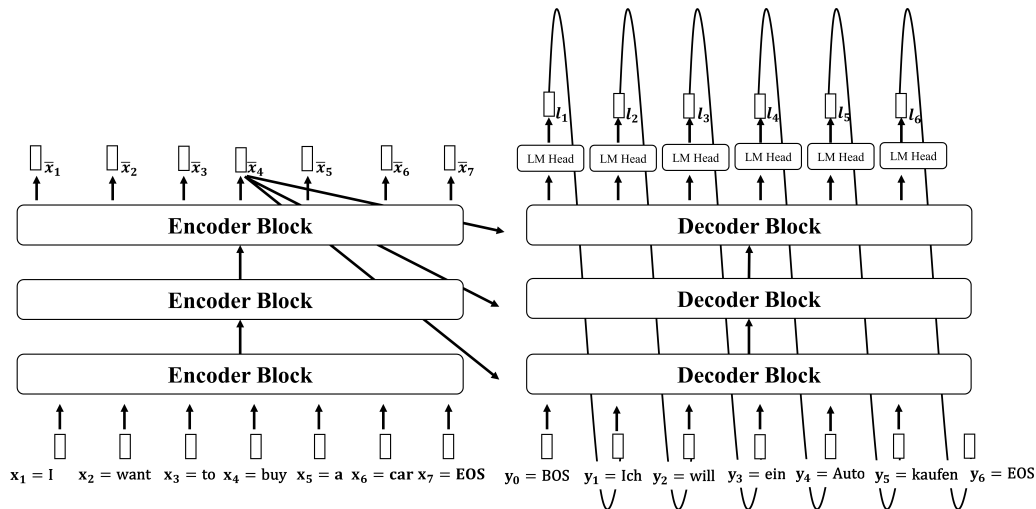
Abbildung 4.5: Vereinfachter Aufbau eines Transformers (Platen, 2020)
